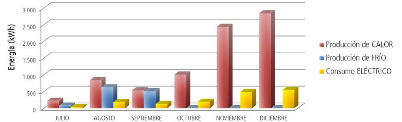
Datos reales extraídos del Easynet de las bombas de calor desde su instalación
