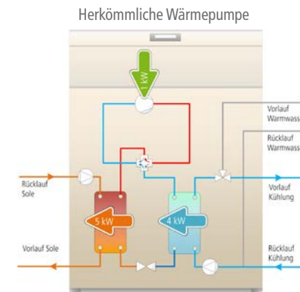
Herkömmliche Wärmepumpe
