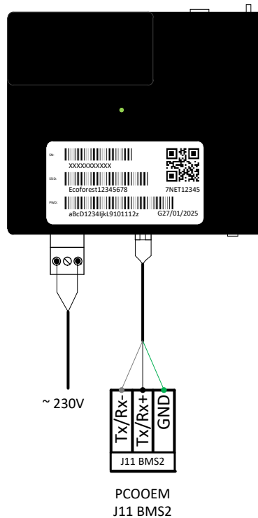
Figura 3.1. Instalación del GATEWAY EASYNET G2 al equipo ECOFOREST.
