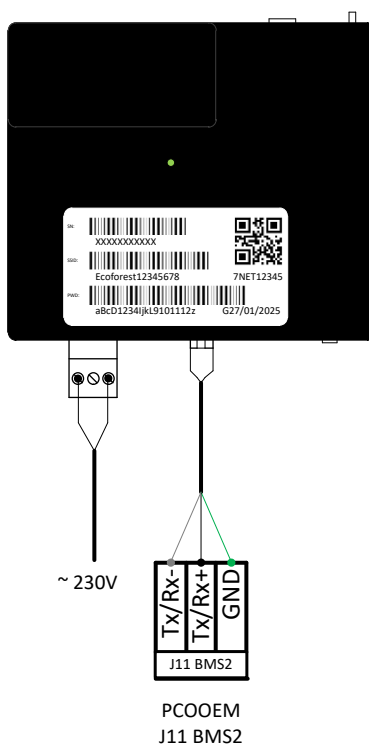
Afbeelding 3.1. Installatie van GATEWAY EASYNET G2 op het ECOFOREST-apparaat.
