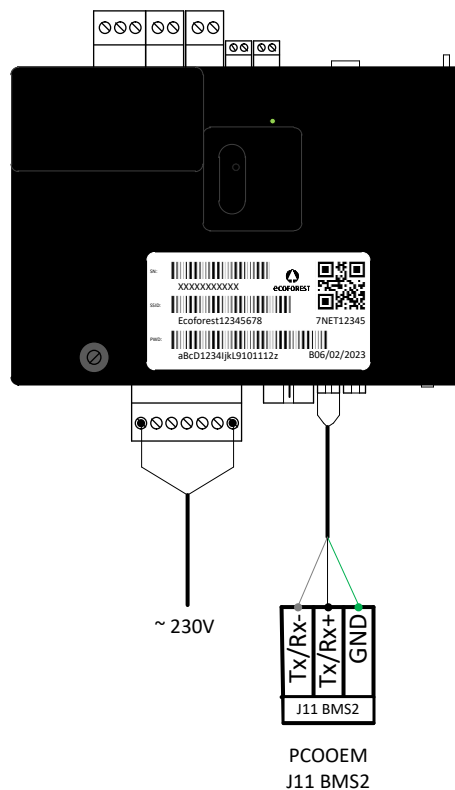
Figura 3.1. Instalación del GATEWAY EASYNET al equipo ECOFOREST.
